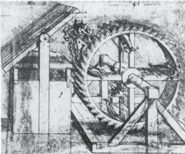
Macchina bellica. Le quattro balestre scaricano la freccia a ogni quarto di giro della ruota.
